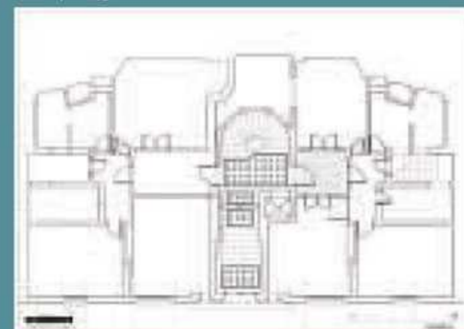
Κάτοψη κτηρίου Ζαλοκώστα 7, Φ. Μπέλλιου, Φ. Κανελλοπούλου
